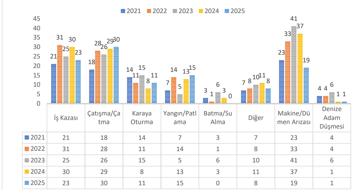
Şekil 2 2021-2025 takvim yıllarında meydana gelen kaza/olayların türüne göre dağılımı
