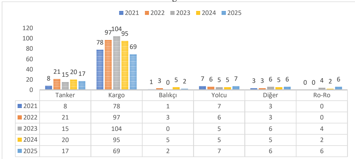
Şekil 3 2021-2025 takvim yıllarında meydana gelen kaza/olayların gemi tipine göre dağılımı
