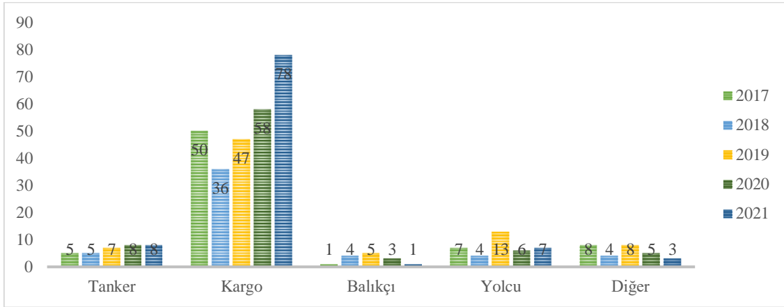
Grafik 3: 2017-2021 Yılları Arasında Meydana Gelen Kazaların Gemi Tipine Göre Dağılımı
