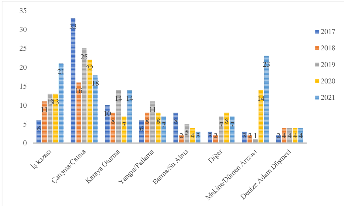
Grafik 2: 2017-2021 Yılları Arasında Meydana Gelen Kazaların Kaza Türüne Göre Dağılımı
