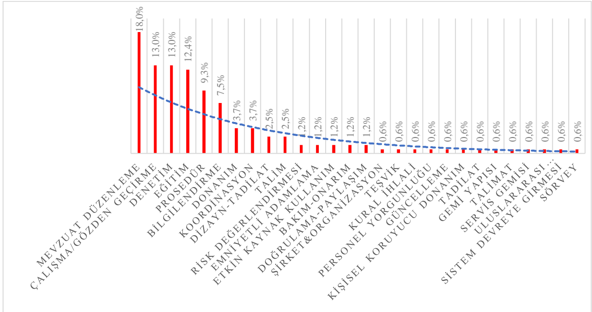
Grafik 8: 2017-2021 Yılları Arasında İncelemesi Yapılan Kazalarda Tavsiyelerin Kategorik Dağılımı
